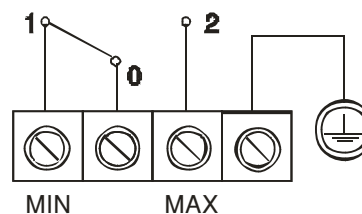
Šema elektropovezivanja
